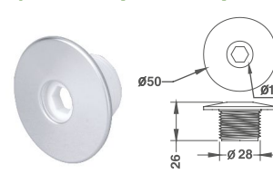
φ2" Face (Standard) Jet
