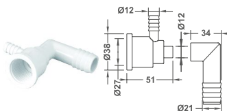
L-Type Jet Body
